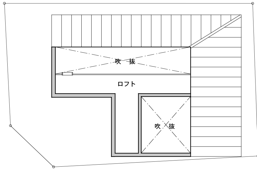
ロフト階平面図
