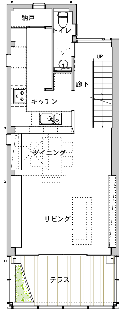
2階平面図
