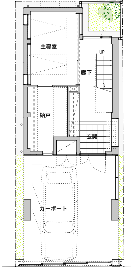
1階平面図
