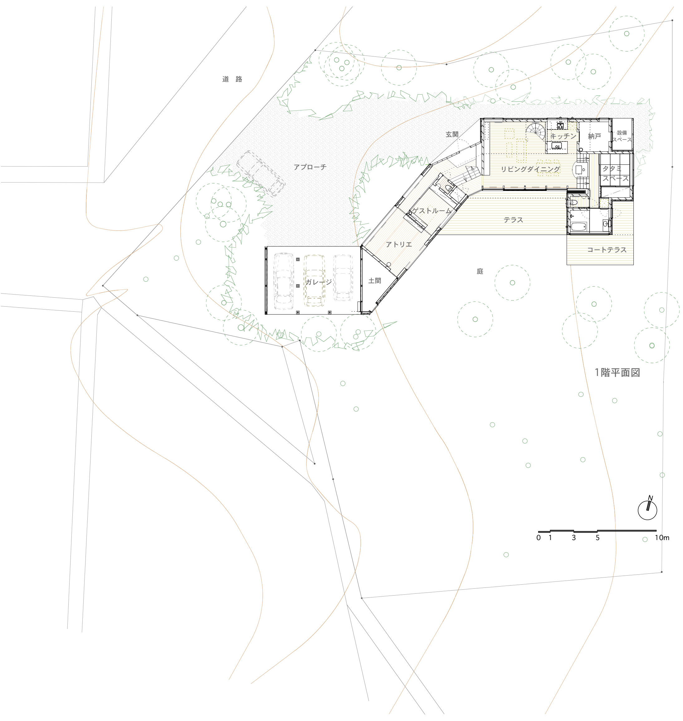
2階平面図
